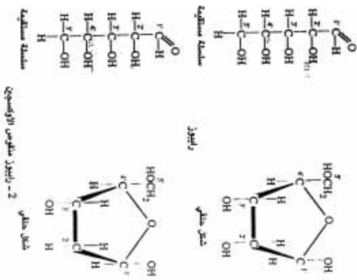
الشكل رقم (٩) التركيب الكيميائي لنوعي السكر الخماسي
